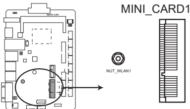
Apollo Lake mSATA / Mini PCIe x1 slot
