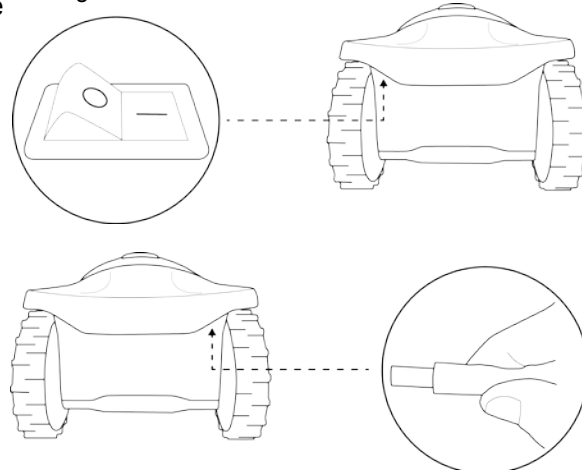
Veiligheidsschakelaar
