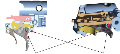
Birinci aşama ayar vidası İkinci aşama ayar vidası
