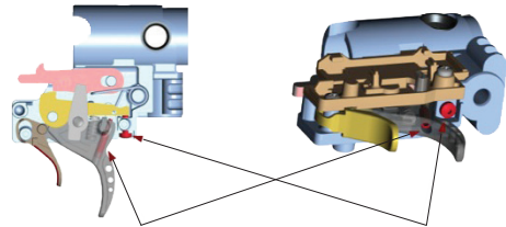
Stellschraube erste Phase Stellschraube zweite Phase
