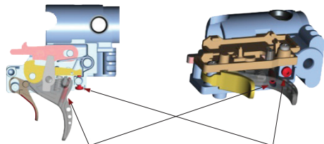
Винт регулирования первой ступени
