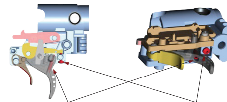
Ensimmäisen vaiheen säätöruuvi
