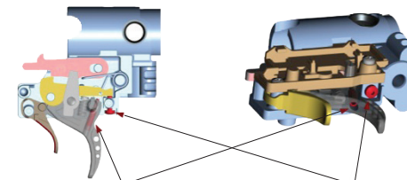
Tornillo de ajuste del primer tiempo
