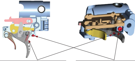
Βίδα ρύθμισης πρώτου σταδίου Βίδα ρύθμισης δεύτερου σταδίου
