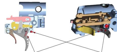
Vite di regolazione di primo tempo
