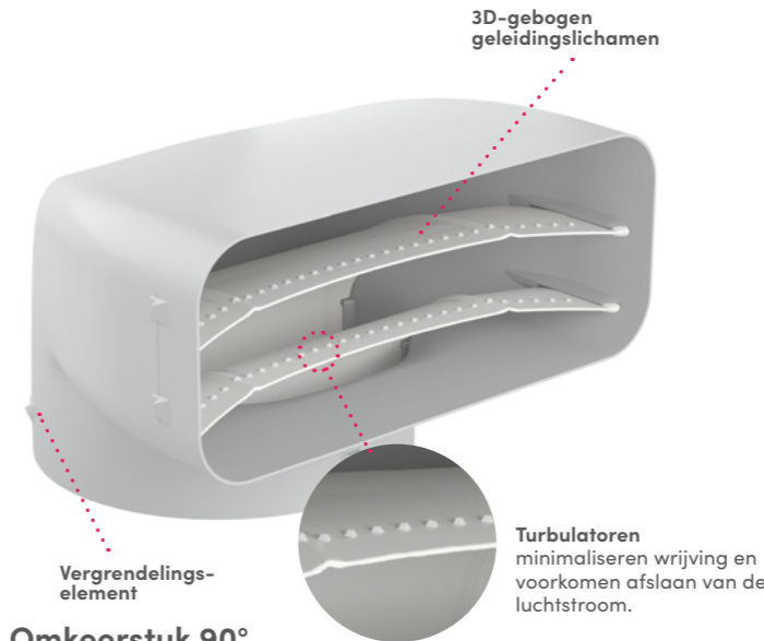
Omkeerstuk 90° P-UR 150
