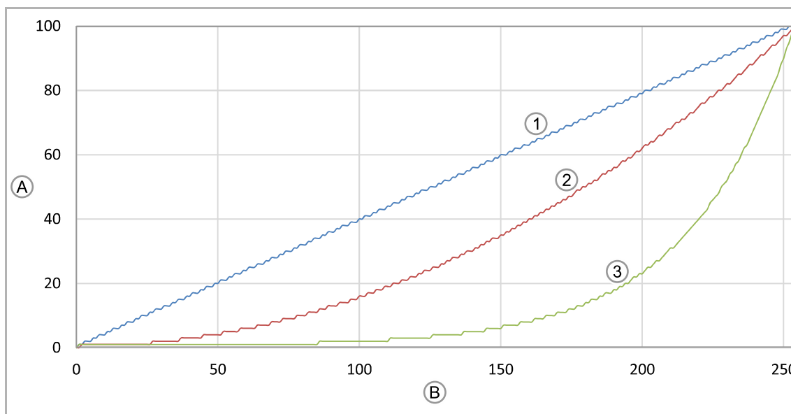
Afb. 8: Vergelijking dimcurve
