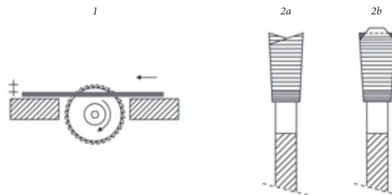
fig 8. 1. Instelhoogte – 2a. Wisseltand – 2b. Trapezium-vlaktand
