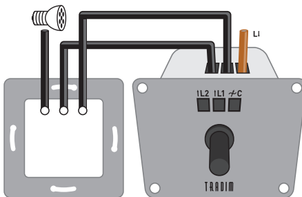
Schakelaar 1
