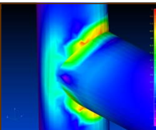
Weergave van de optredende afschuifspanningen onder invloed van belastingssituatie 5
