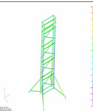
Weergave van de optredende spanning onder invloed van belastingssituatie 3
