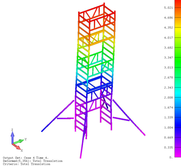
Figuur 2: Weergave optredende vervormingen
