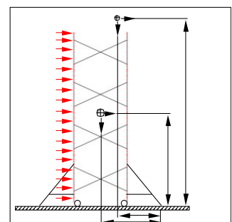
Longitudinaal - Outdoor
