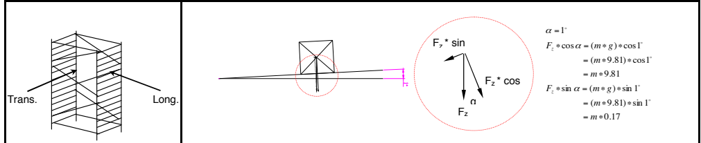
Figuur 1: Combinatie van belastingen volgens NEN-EN 1004:2004
