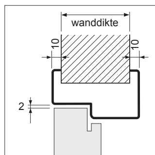
bovendorpel profiel stompe uitvoering deurdikte 54 mm
