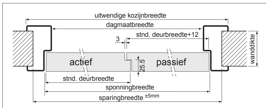
horizontale doorsnede MonoPlus stompe uitvoering, sponning/contra-sponning
