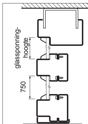
verticale doorsnede, zijlicht opdekuitvoering
