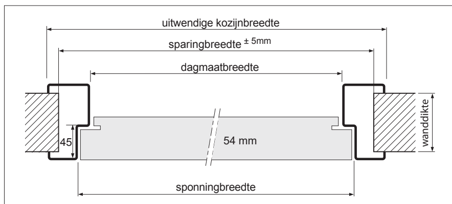
horizontale doorsnede MonoPlus stompe uitvoering, deurdikte 54 mm
