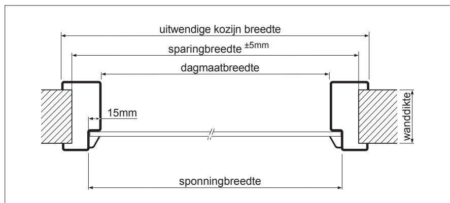
horizontale doorsnede raamkozijn
