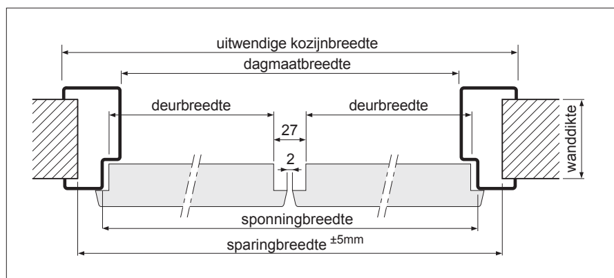
horizontale doorsnede MonoPlus opdekuitvoering
