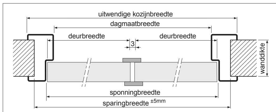
horizontale doorsnede MonoPlus stompe uitvoering met aanslaglatten
