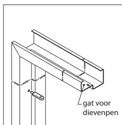
bevestiging deurpanelen, draagclip voor stompe panelen
