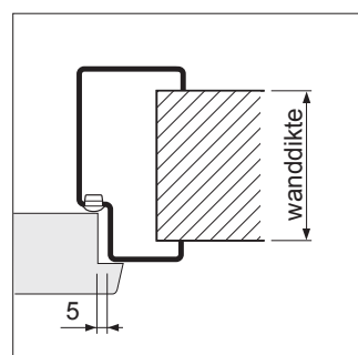
profiel opdekuitvoering
