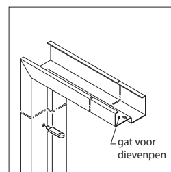
bevestiging deurpanelen, draaglip voor stompe panelen
