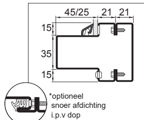
pui-kalfdeel 45x15 mm of 25x15 mm
