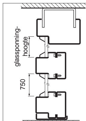
verticale doorsnede, zijzicht opdekuitvoering
