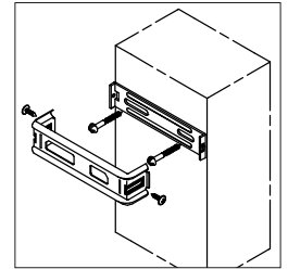
wandbevestiging muurbeugel Mono
