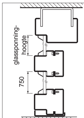
verticale doorsnede, zijlicht opdekuitvoering
