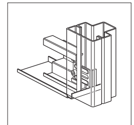
verbinding grondregel met puistijl
