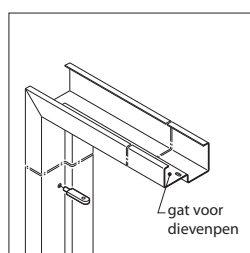
bevestiging deurpanelen, draagclip voor stompe panelen
