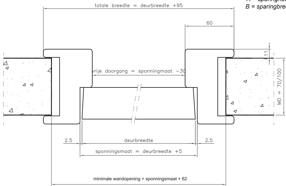
horizontale doorsnede houten kozijn stomp
