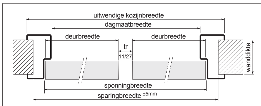
horizontale doorsnede MonoPlus stompe uitvoering
