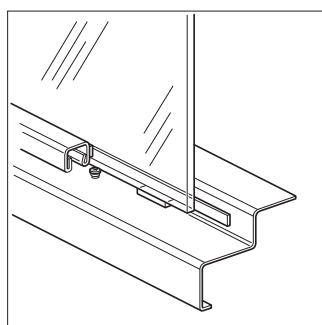
stalen glaslijst 15x15 mm t.b.v. sponning 25x15 mm
