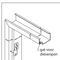
bevestiging deurpanelen, draagclip voor opdekpanelen
