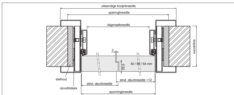
horizontale doorsnede DuoFlex stompe uitvoering sponning/contra-sponning
