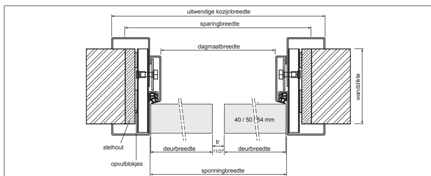
horizontale doorsnede DuoFlex stompe uitvoering
