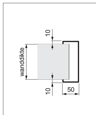
wandbeëindigingsprofiel met Mono-muurbeugel
