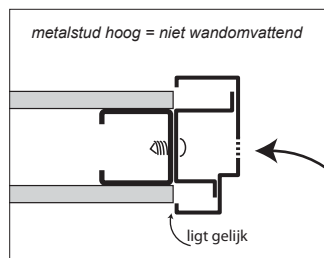
metalstud, met gaten als de gipsplaten al zijn geplaatst
