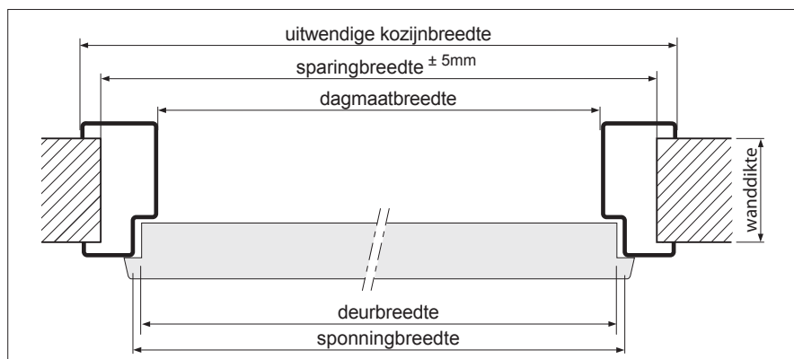
horizontale doorsnede MonoPlus opdekuitering
