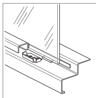
stalen glaslijst 28x15 mm t.b.v. sponning 45x15 mm
