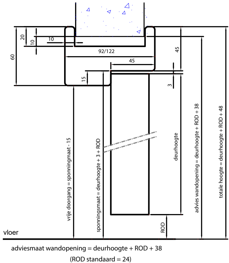
verticale doorsnede, stomp
