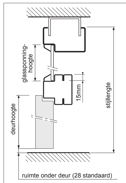
verticale doorsnede met bovenlicht en vaste bovendorpel, opdekuitvoering
