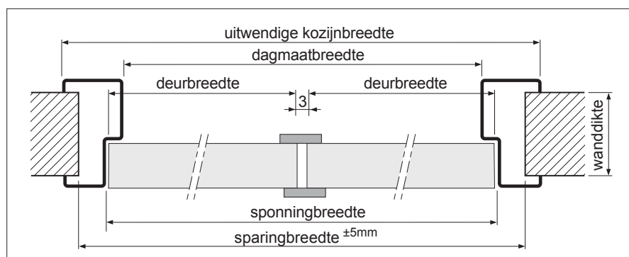
horizontale doorsnede MonoPlus stompe uitvoering, sparring/contra-sparring ook voor brandwerende combinaties
