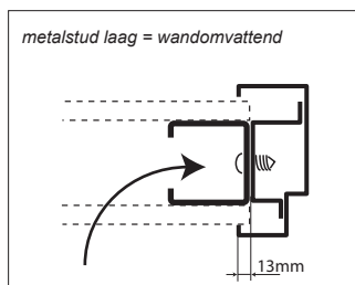
metalstud, laag, zonder gaten gipsplaten worden later geplaatst
