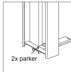
standaard stelstripdetail
