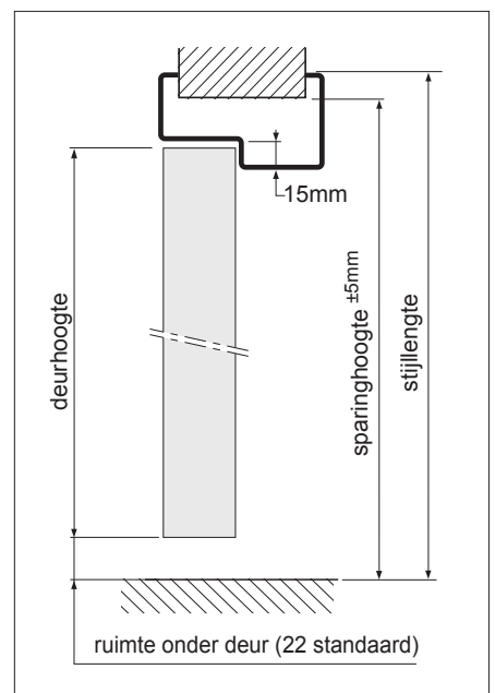
verticale doorsnede, stompe uitvoering
