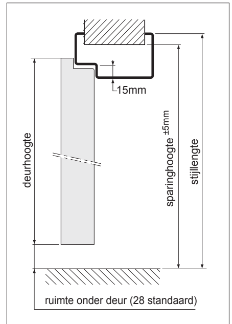
verticale doorsnede, opdekuitvoering
