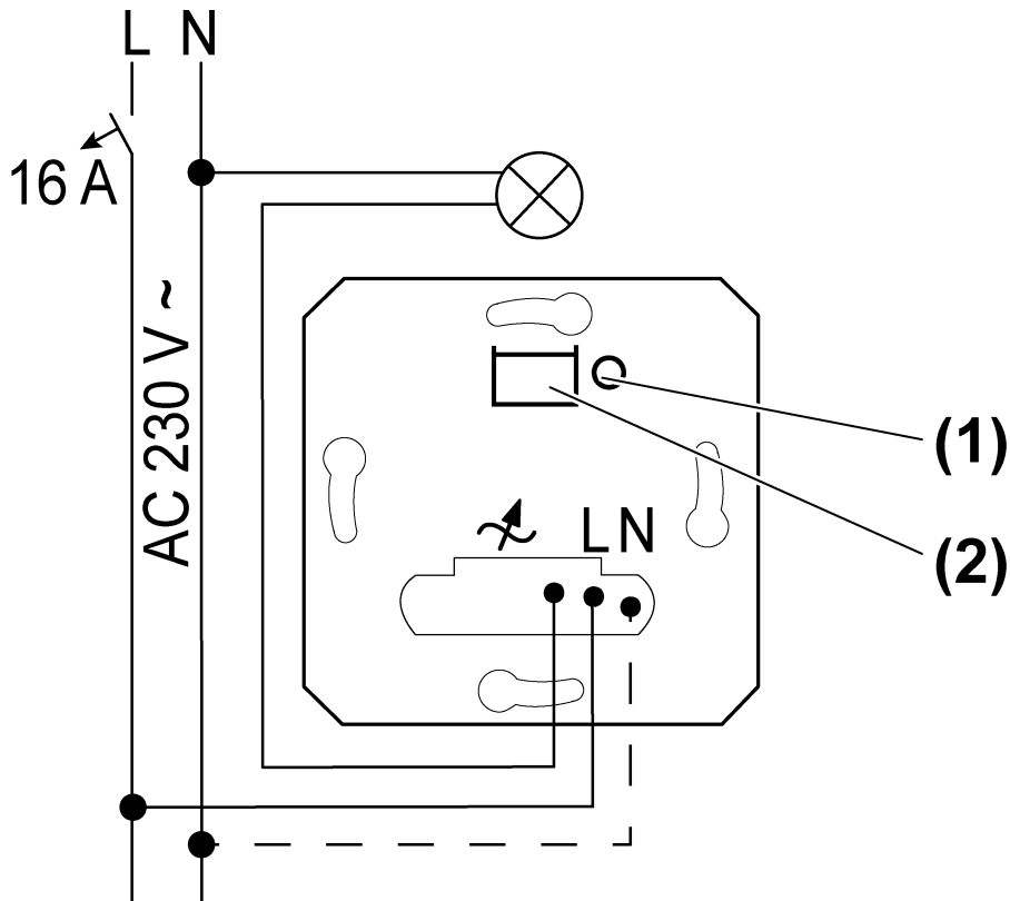
Afbeelding 1: Aansluitschema
