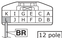
0914-211 FRONT DOOR LATCH AND LOCK ACTUATOR (LH)
