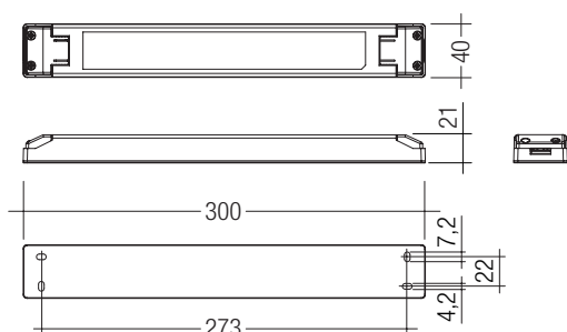
LCU 96W 24V SR TOP
