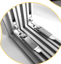
claplock corner connector 100er profile Art. : 60188
