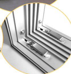
claplock corner connector 150er profile Art. : 60222
