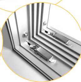
claplock corner connector 150er profile Art.: 60222
