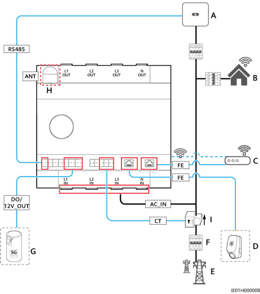
Abbeelding5-2 Kaart voor kabelaansluiting: externe Ct-aansluiting (stroomsterkte > 63 A)
