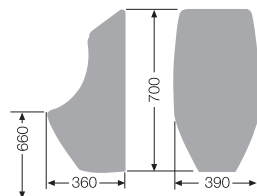
Model keramischcompact
