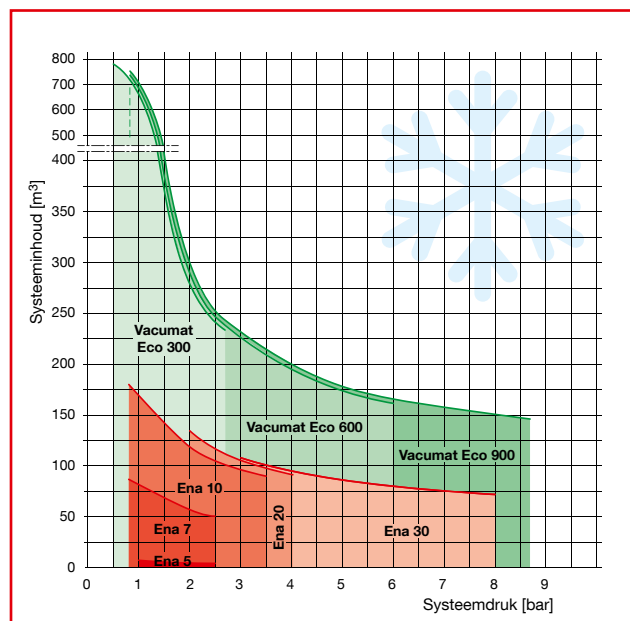
Selectiegrafiek voor koeling
