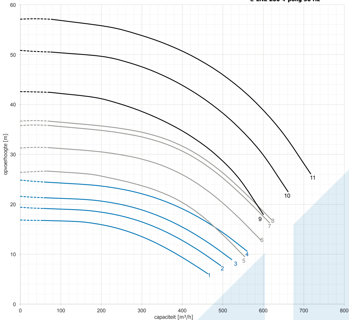
e-LNE 200 4-polig 50 Hz
