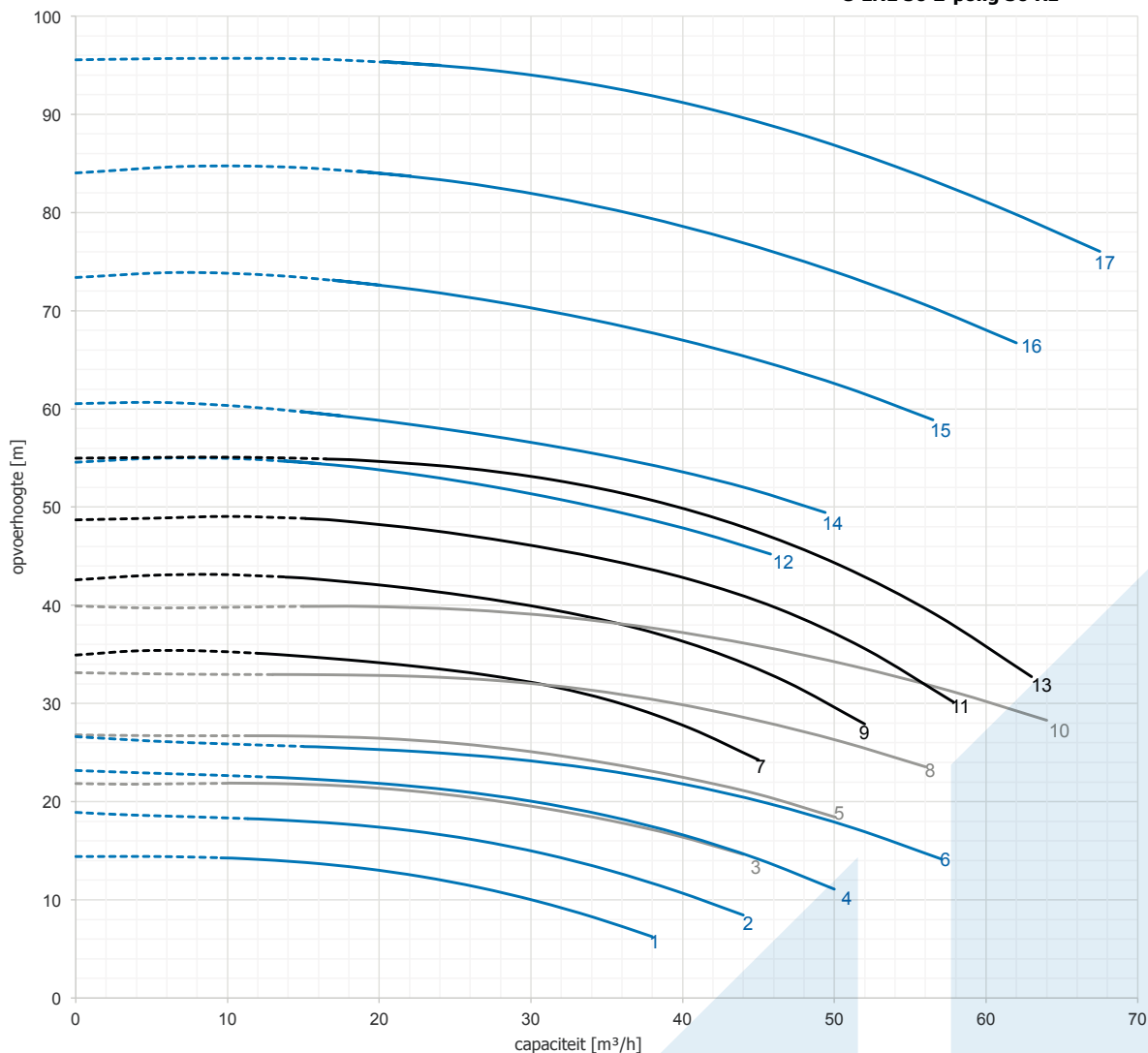
e-LNE 50 2-polig 50 Hz
