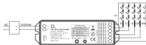
Anschluß von LED-Leiterplatten RGB+CCT
