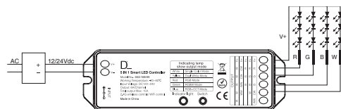
Anschluß von LED-Leiterplatten RGBW
