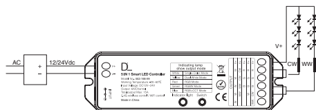
Anschluß von LED-Leiterplatten TUNEABLE WHITE
