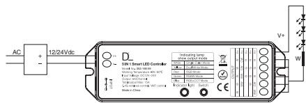
Anschluß von einfarbigen LED-Leiterplatten
