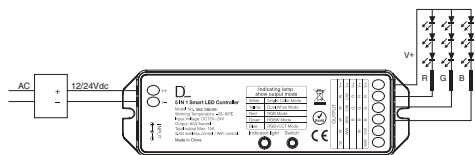
Anschluß von LED-Leiterplatten RGB
