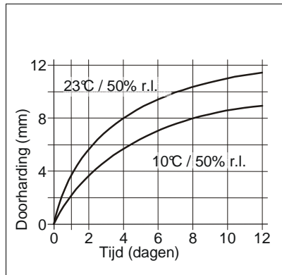
Schema 1: Uithardingstijd voor Sikaflex®-290 DC
