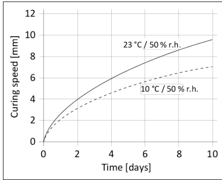
Schema 1: Doorhardingssnelheid Sikaflex®-508
