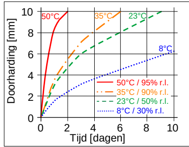
Schema 1: Doorhardingssnelheid voor Sikasil® AS-70
