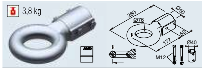
Occhione NATO N76/E Cod. art. 1 224 666
