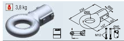
Occhione Francia F68/E1 Cod. art. 1 224 665
