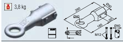
Occhione Inghilterra E40/A Cod. art. 1 224 662
