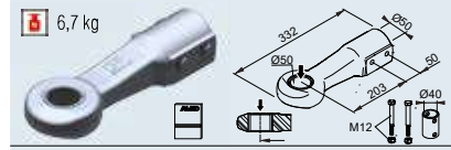
Occhione DIN D50 / D40 Cod. art. 1 730 611
