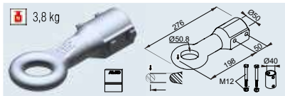
Occhione Inghilterra E50/A Cod. art. 1 224 664
