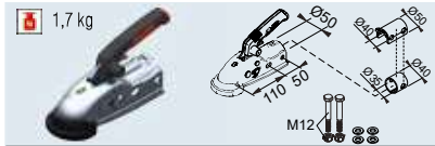
Giunto a sfera AK161 Ø35-Ø50 Cod. art. 1 730 806
