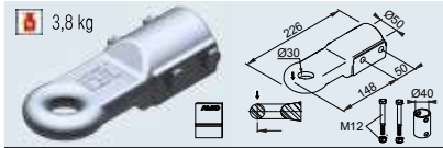
Occhione Inghilterra E30/A Cod. art. 1 224 661
