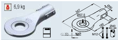
Occhione Svezia VBG 57,5 Cod. art. 1 225 125
