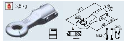
Occhione DIN D40/F Cod. art. 1 224 660
