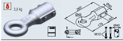
Occhione Italia I45/F Cod. art. 1 224 663
