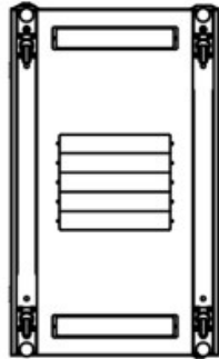
Unteransicht
