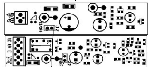
J2 INSERITO: 12V ac/dc J2 NON INSERITO : 24V ac/dc
