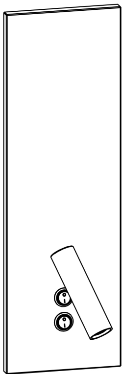
L440×W140×H90(mm) LED-3+4W
