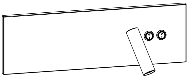
L440×W140×H90(mm) LED-3+4W
