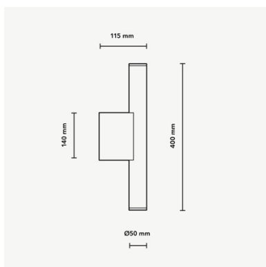
DIMENSIONS
