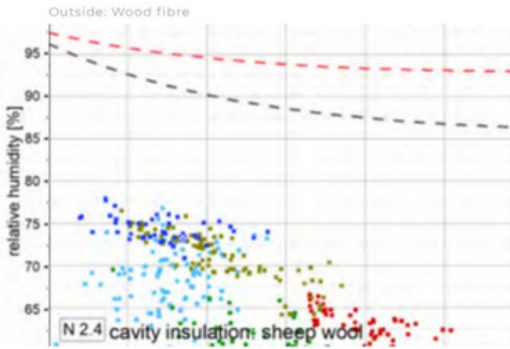
De metingen uit de 'point cloud' laten zien dat schapevoolisolatie ruim onder de aanbevolen grenscurves blijft. (© Fraunhofer Institute for Building Physics / Holzforschung Austria 2023)
