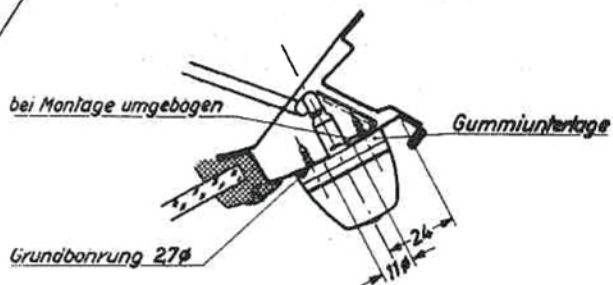
Schnitt A-B (nach Fertigmontage der Antenne)
