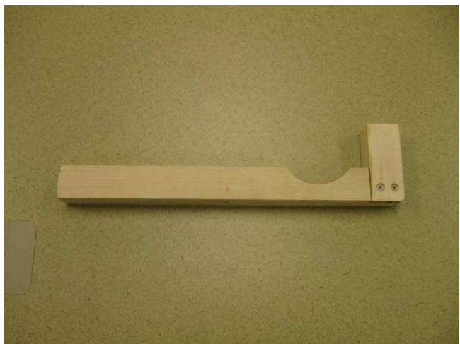
Illustration 101 - Sostenuto lever
