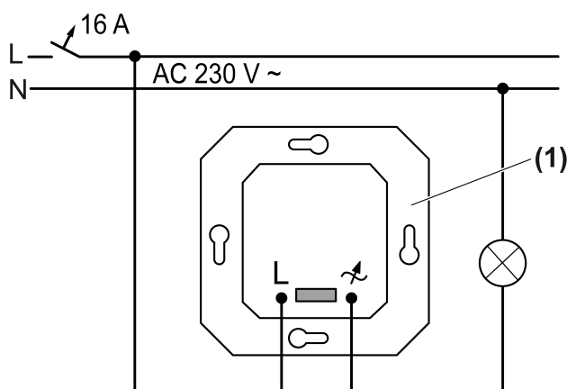
Afbeelding 2: Aansluitschema
