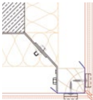
UITSPRINGENDE HOEK ZONDER PROFIEL
