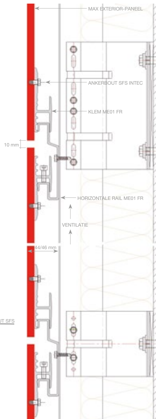
VERTICALE DOORSNEDE HORIZONTALE VOEG
