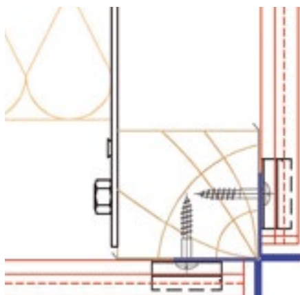
UITSPRINGENDE HOEK MET KRUISVORMIG PROFIEL
