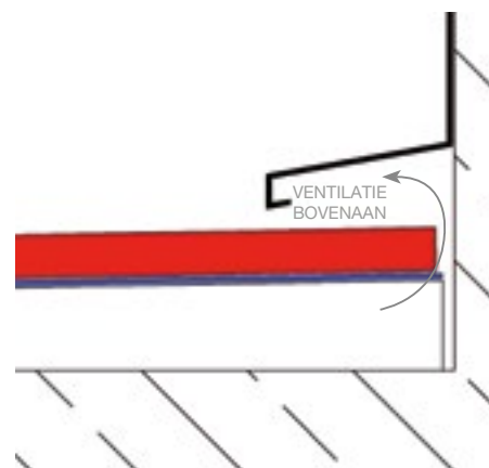
VERTICALE DOORSNEDE VAN HET PRINCIPE VAN DE VERBINDING MET DE GEVEL
