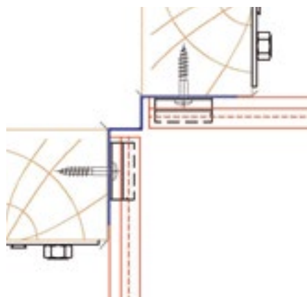
INSFRINGENDE HOEK MET HOEKPROFIEL
