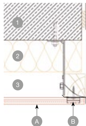
VENSTERDORPEL
