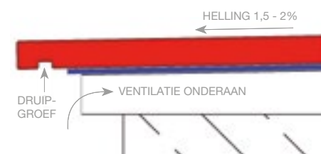
DETAIL VAN HET PRINCIPE VOOR DRUIPGROEF, VENTILATIE EN HELLING
