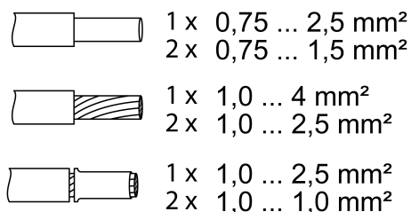
Afbeelding 2: Klembare leidingdoorsnedes
