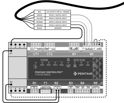
Abbildung 6: ControlPro Verdrahtungsdiagramm
