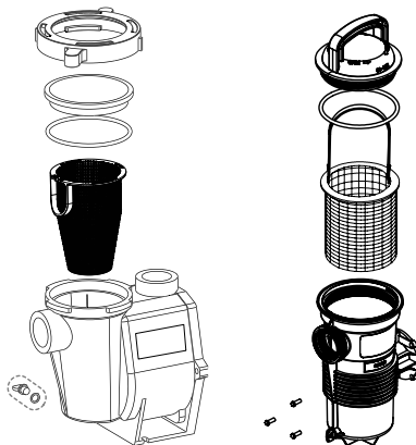
Whisperfilo VS2
