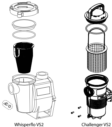
Gruppo prefiltro
