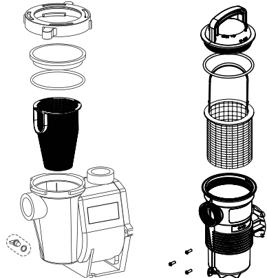
Whisperflo VS2
