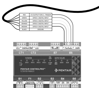
Figura 6: diagramma di cablaggio di ControlPro+
