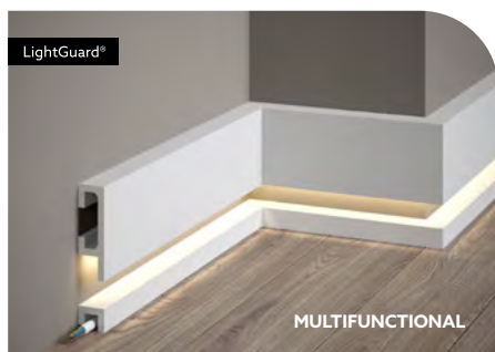
QL019 + QL021 mat QL019P + QL021P satin (RAL9003) PolyForce® | ScratchShield® QL019 200 x 8 x 2,5 cm QL021 200 x 2 x 2,5 cm
