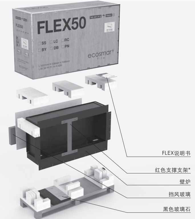
壁炉包装 *不适用于Flex Bench型号产品。
