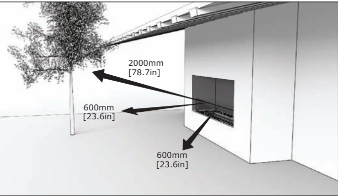
户外间距（需涵盖屋檐以确保雨水不会浸湿燃烧器。与当地政府核实是否安装环境在政府的认证编号里。）
