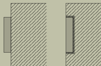
Dimensioni foro per incasso L.625 x P.135 x H.426 mm
