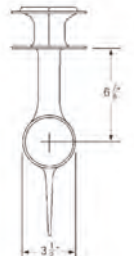
Vista posterior Rear View Vista posteriore
