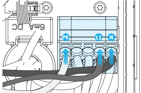
Figuur 5: Elektrische aansluiting, S-line / Pro-line, 1 fase
