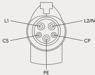
Fahrzeugstecker - Typ 1
