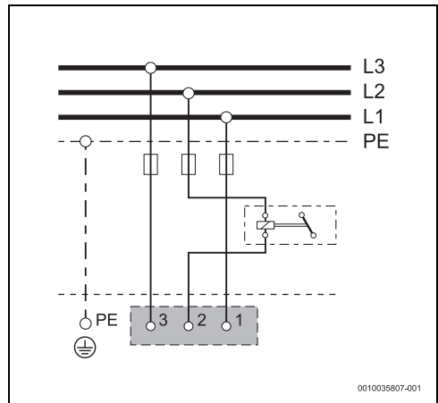
Rys. 148 Schemat elektryczny
