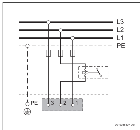
Bild 40 Schaltplan
