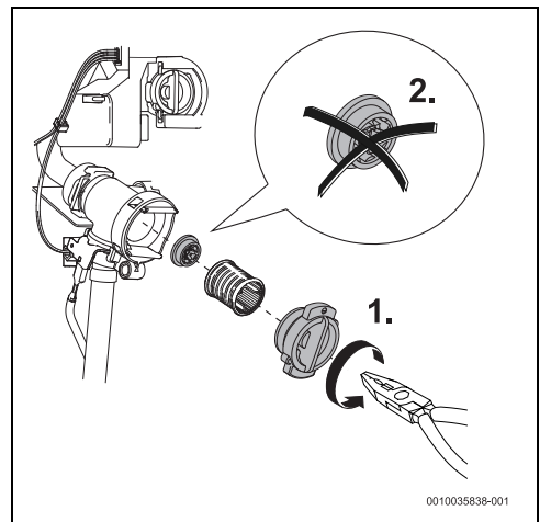
Rys. 163 Usuwanie ogranicznika przepływu.
