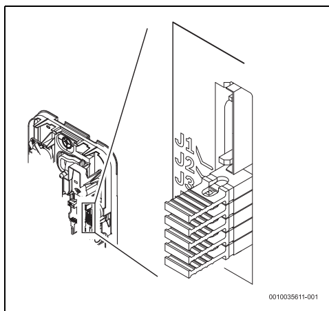
Rys. 146 Dołączone zworki elektroniczne
