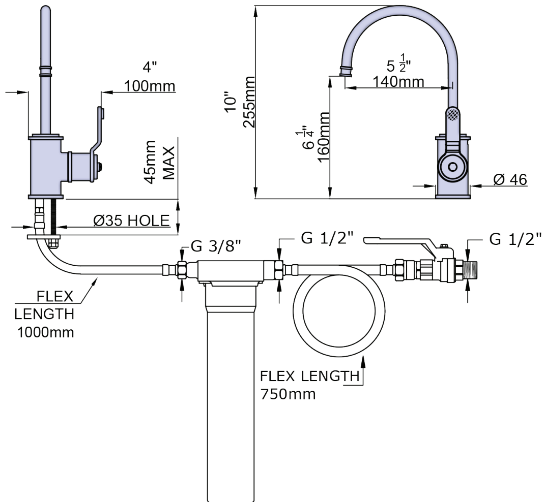
Mini Filtration Tap
