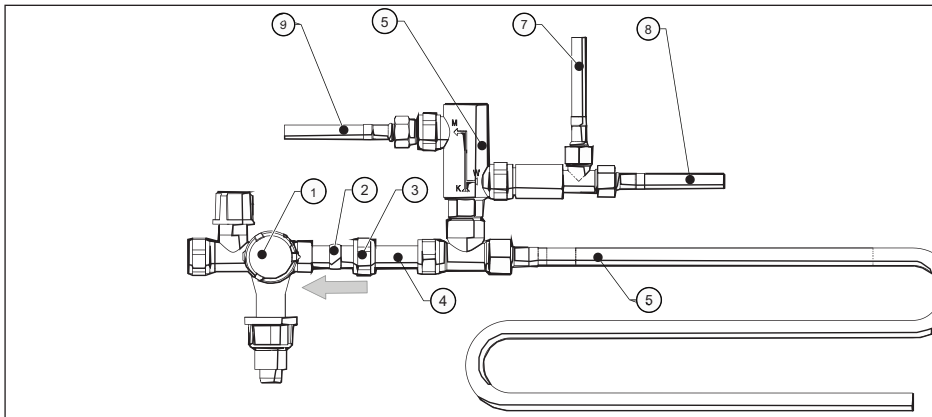
Fig 2 Overzicht aansluitingen
