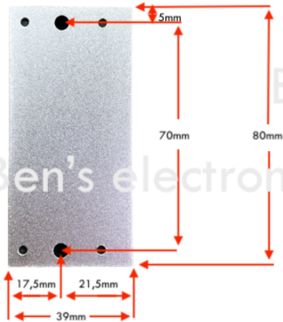
Achterkant Magneet
