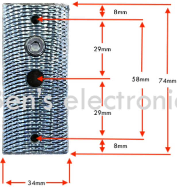
Achterkant Magneet
