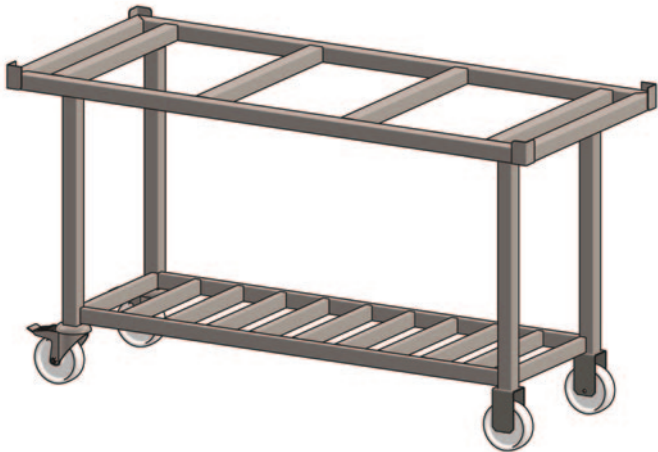
Typ TPP-H | H-Verstrebung
