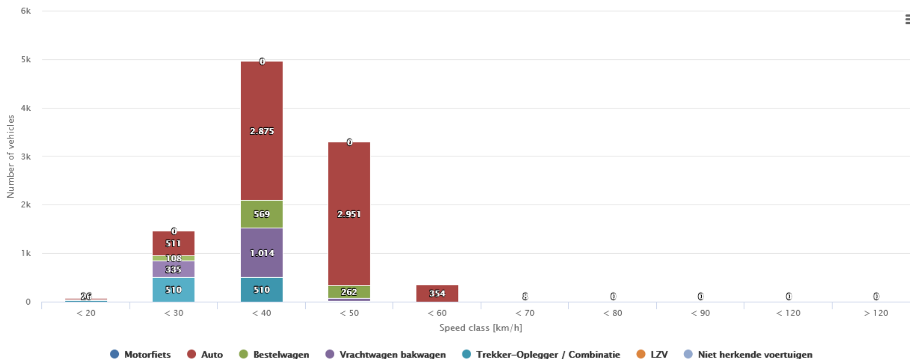
Grafiek 1: Frequentie – verdeling van voertuigcategorieën naar snelheidsklassen in de periode van 10.06.2021 17:00 tot 10.07.2021 17:00
