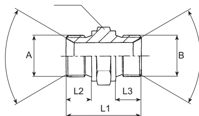
44 A..BM..BM : ADAPTEURS DROITS MALES Filetage : B.S.P. cylindrique
