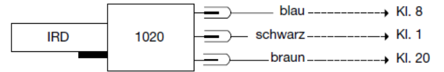
IRD ANSCHLUSS
